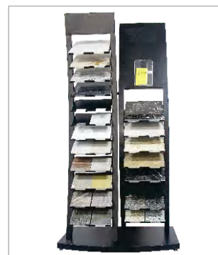
VQ137 Sample size: 6" x 12"/12" x 12" Capacity: 20/40Pcs
